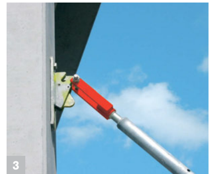
3 Zeitersparnis bei der Montage der Strebe am Fertigteil durch zeitsparenden Schnellverschluss.
