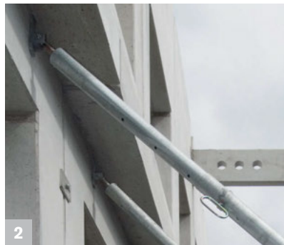
2 Schnellere Längeneinstellung durch Grob- und Feinjustierungsmöglichkeit.
