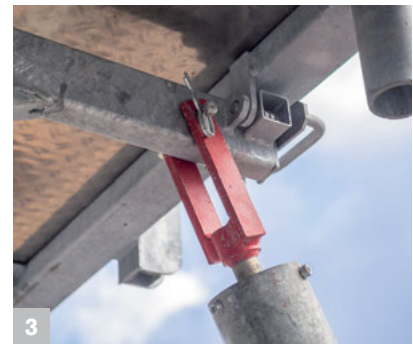
3 Anschlussmöglichkeit für Richtstreben.
