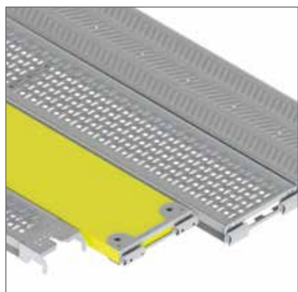
► Kompatibel mit allen Hünnebeck Systembelägen
